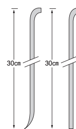
防汚抗菌 ワイド巾木断面図 (Rアリ) (Rナシ) WTH300 WTH300RN
